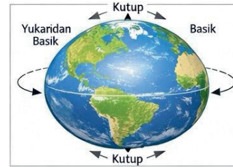
Şekil 2. Dünya’nın Şekli: Basık Elipsoit Modeli.
