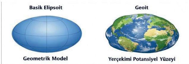
Şekil 1. Basık Elipsoit ve Geoit Karşılaştırması.
